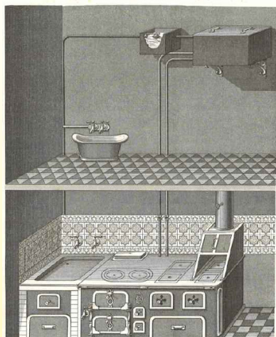
1894 Salle de bain alimentée en eau chaude par cuisinière à bouilleur (Catalogue Chappée, Musée Ultimheat)
