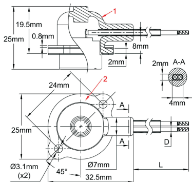
Réarmement automatique
